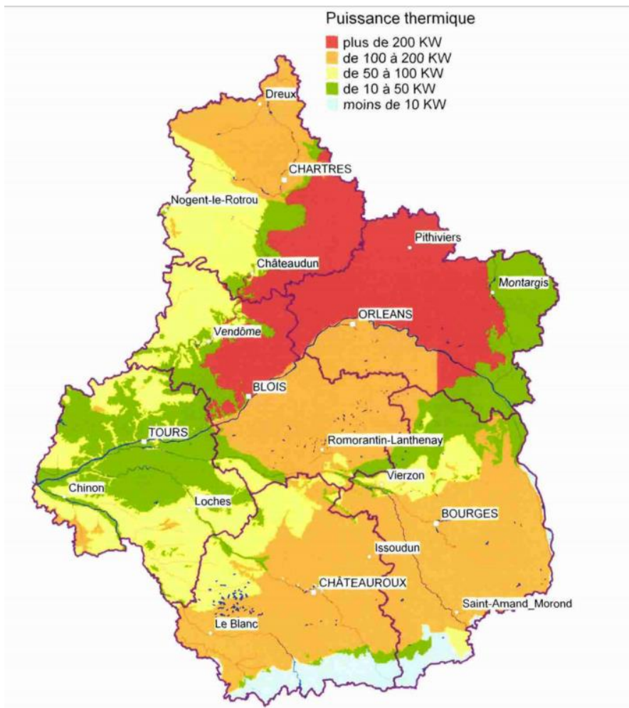
Figure 8 – Puissance thermique disponible dans la nappe - Hypothèse basse, exprimée en KW thermique, pour 6 °C de puisement sur la ressource.
